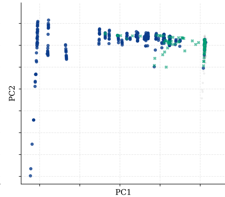
ADASYN
