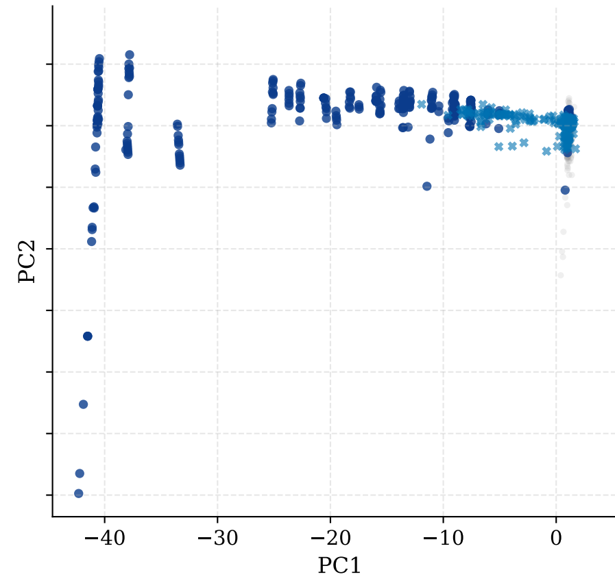
Diffusion (DDPM)
